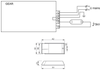
Scheda tecnica Philips HID-PV C 35 /I CDM 220-240V 50/60Hz
